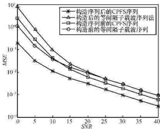
图 2 基本条件下的 2 种特征序列构造前后 MSE 比较
